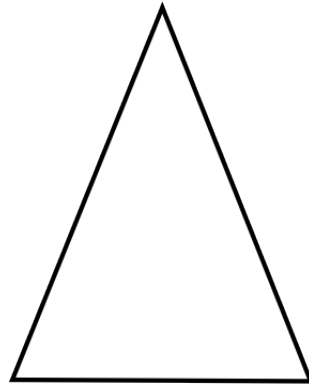
triangle isocèle
